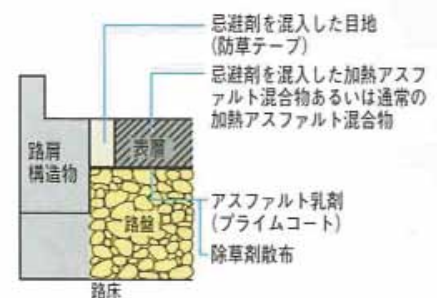
● 防草舗装の概要図
