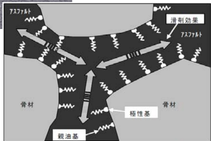
滑剤(界面活性剤)系のメカニズムの概念
