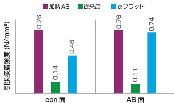
引張接着強度比較図
